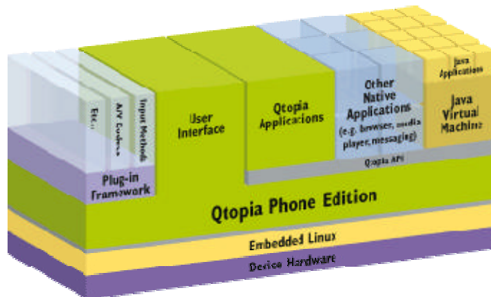
Figure 10: Trolltech Qtopia
